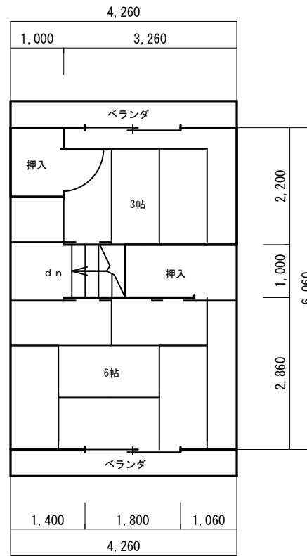
2階平面図
