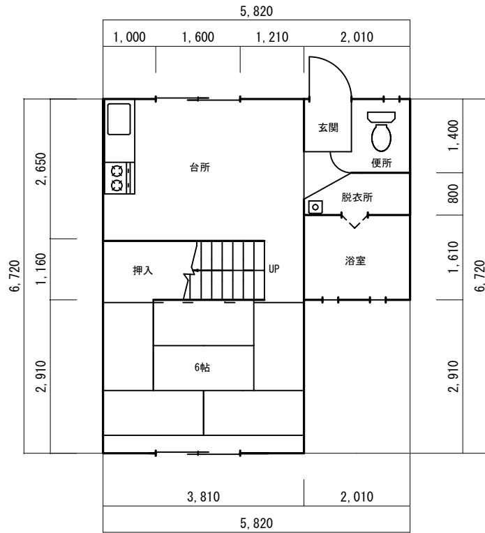
1階平面図
