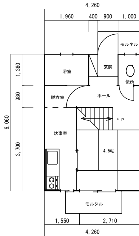
1階平面図
