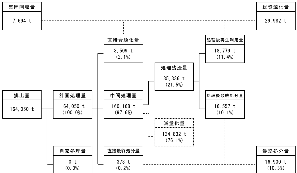
図3 一般廃棄物の排出・処理フロー
