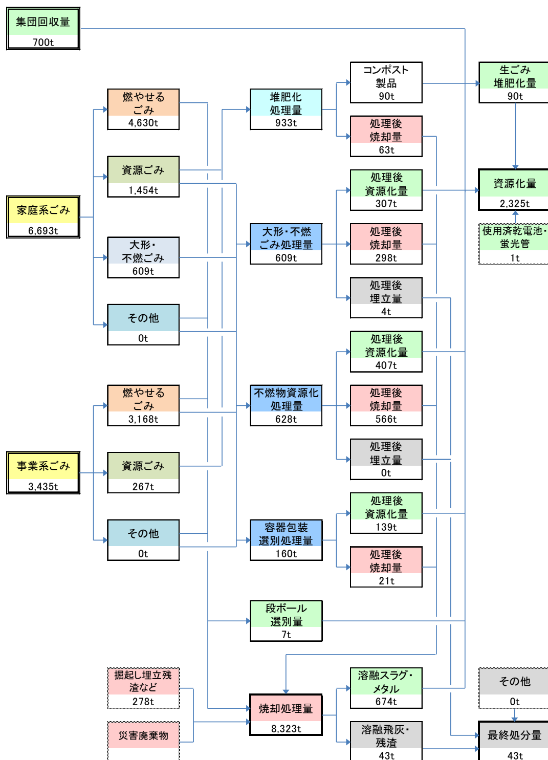
図3.5 ごみ処理フロー(令和元年度)
