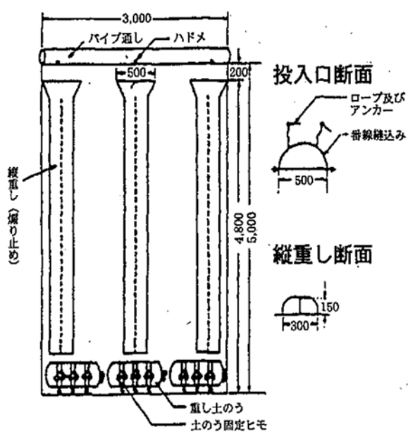
マット標準図（単位：mm）
